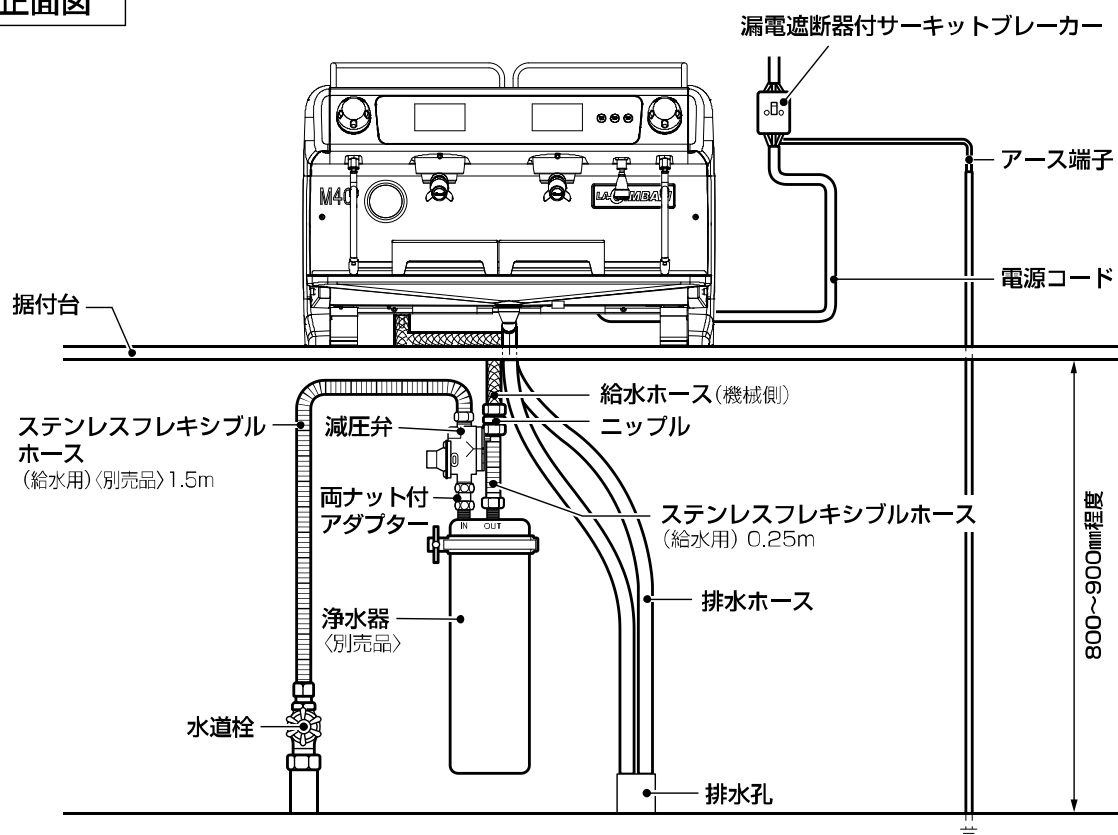
正面図
