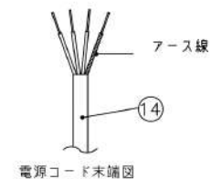
電源コード末端図
