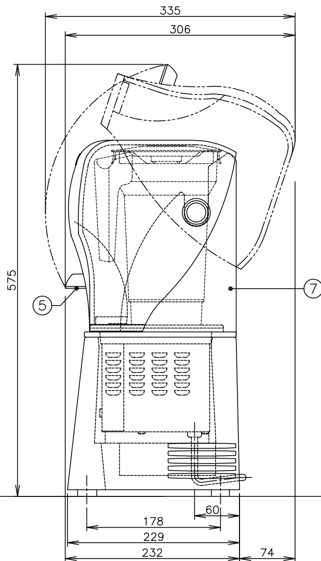
防音フードカバー開時図
