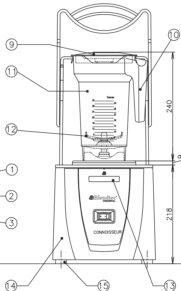
防音フードカバー開時図
