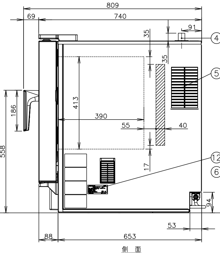
側 面
