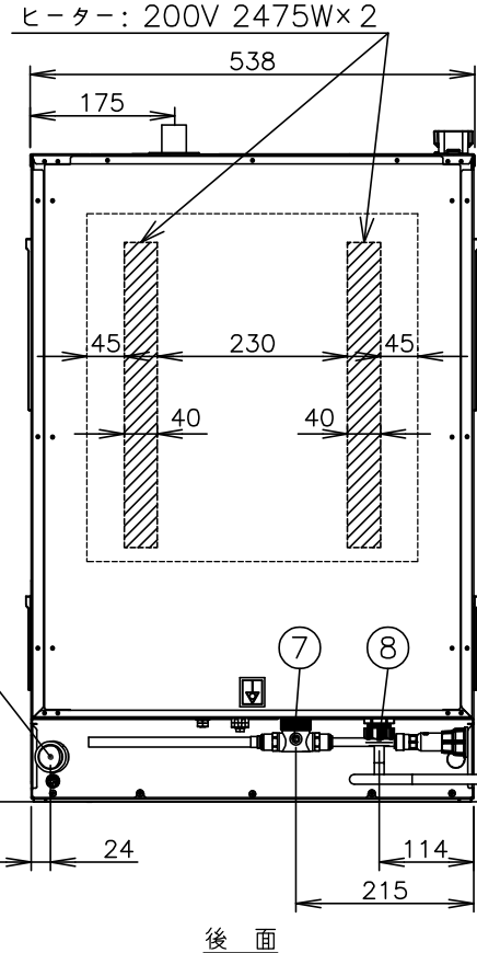
後 面
