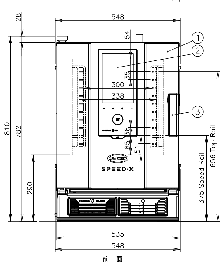
前 面
