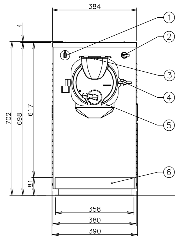
前面
