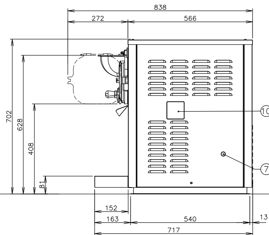
側面
